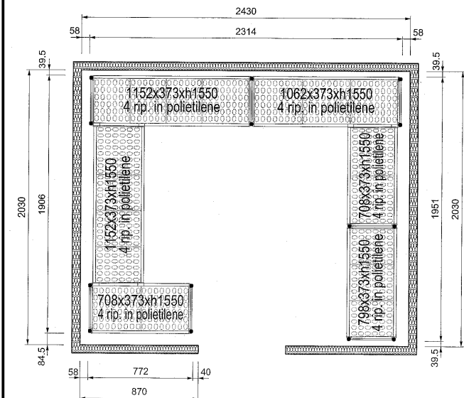
Boven aanzicht
